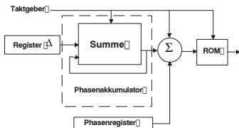
Funktionschema Nr. 1: Direkte Digitalsynthese
