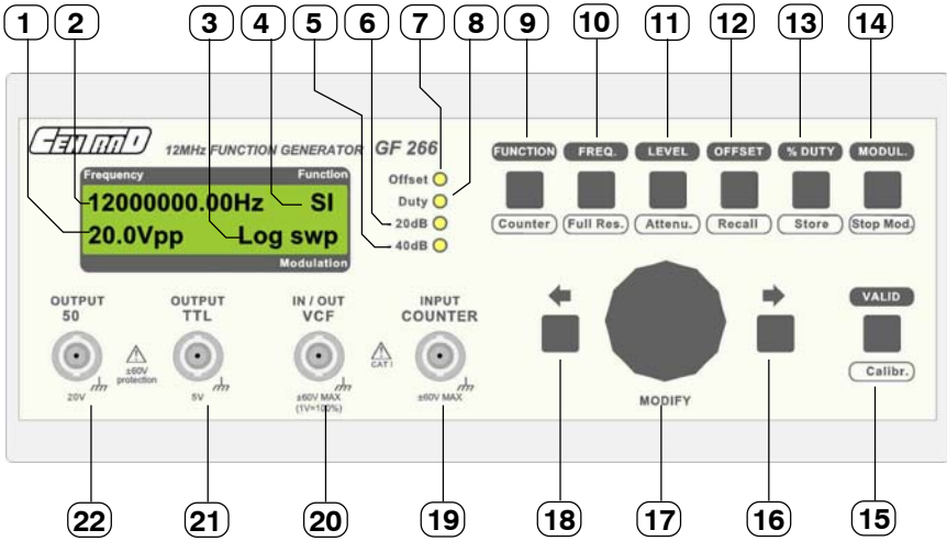
FACE AVANT FRONT PANEL FRONTSEITE
