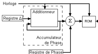
Schéma de principe n° 1 : Synthèse Numérique Directe
